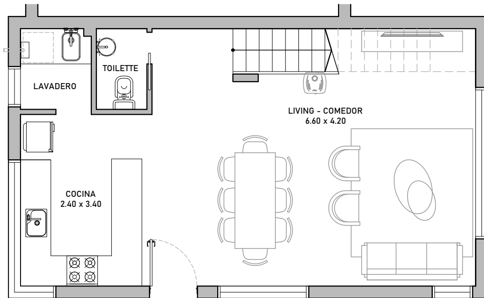
PLANTA BAJA
